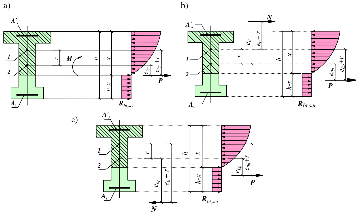
Hình 21 – Sơ đồ nội lực và biểu đồ ứng suất trên tiết diện ngang của cấu kiện khi tính toán theo sự hình thành vết nứt thẳng góc với trục dọc cấu kiện ở vùng chịu kéo do ngoại lực, nhưng chịu nén do lực nén trước a – khi uốn; b – khi nén lệch tâm; c – khi kéo lệch tâm; 1 – điểm lõi; 2 – trọng tâm tiết diện quy đổi
