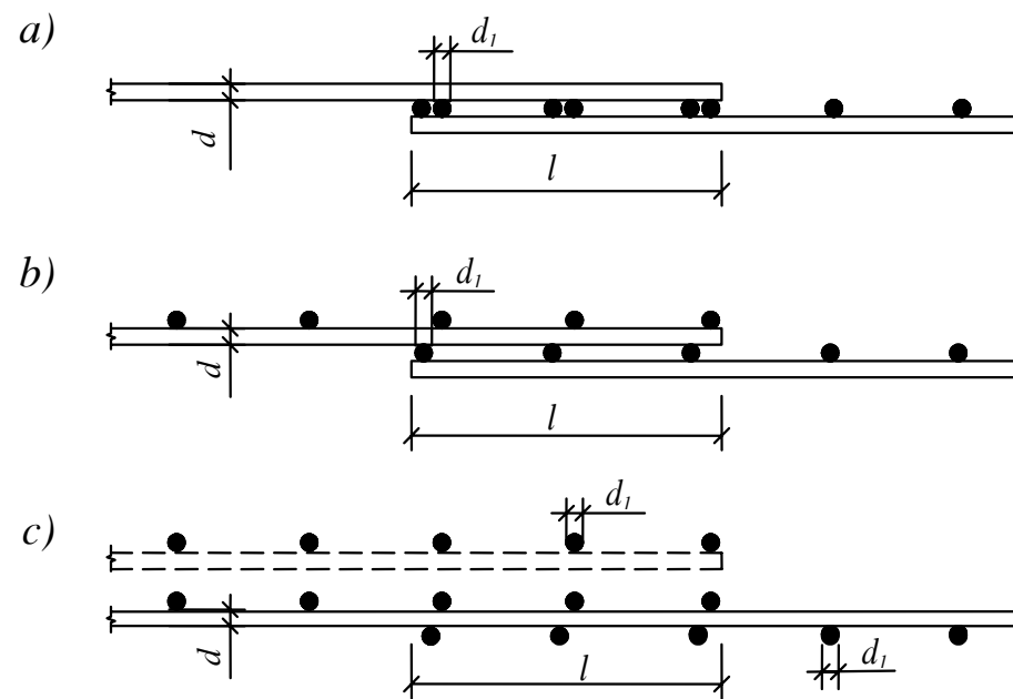
Hình 26 – Nối chồng (không hàn) trong phương chịu lực các lưới hàn làm từ cốt thép tròn trơn
