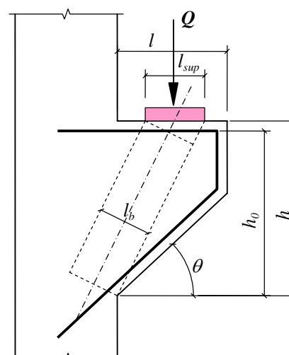
Hình 12 – Sơ đồ tính toán công xôn ngắn
