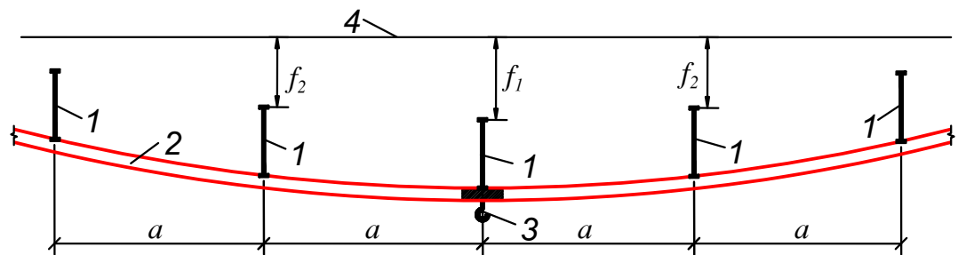
Hình C2 – Sơ đồ để tính độ võng của kết cấu vì kèo khi có đường ray của cầu treo
