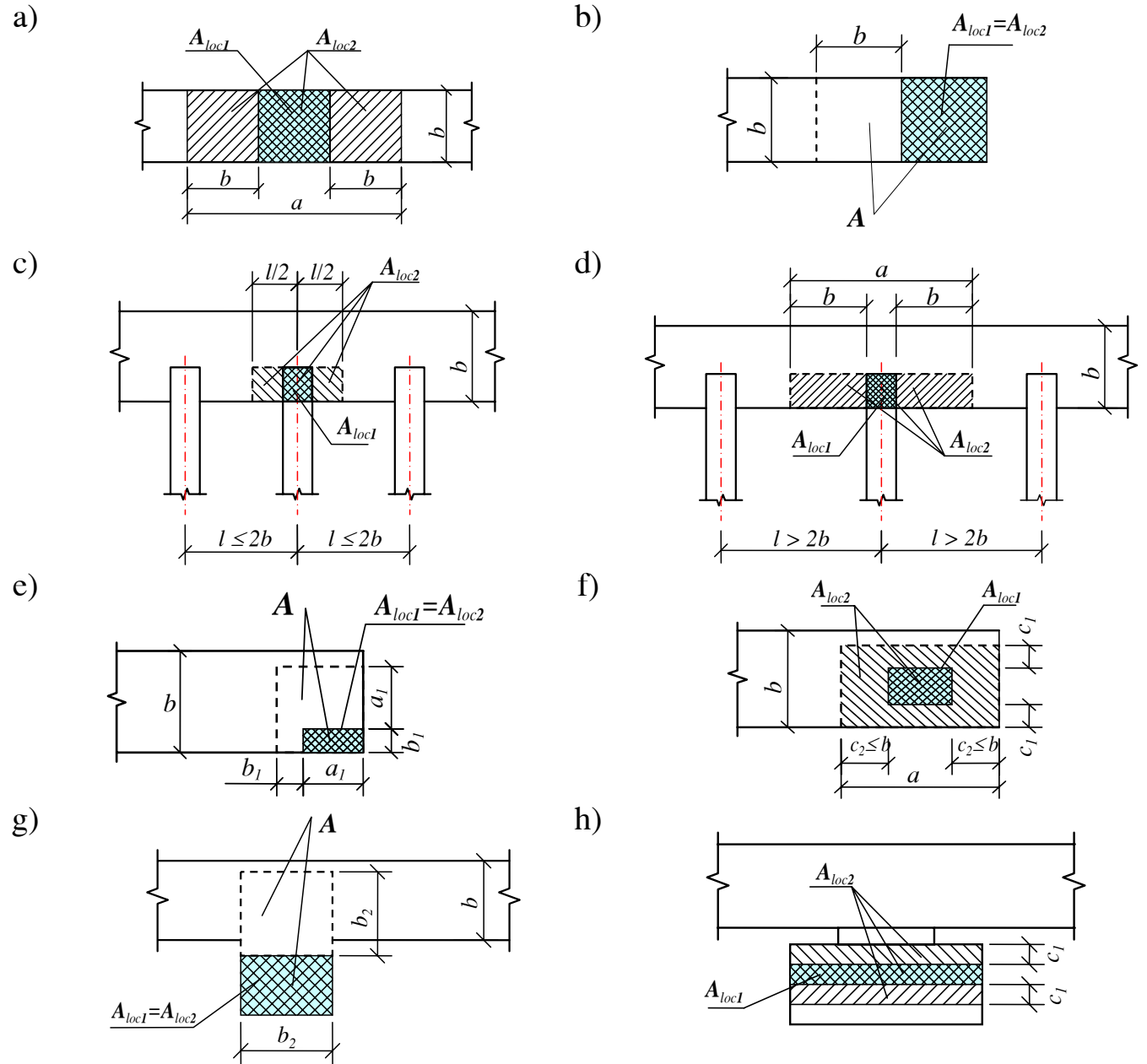
Hình 16 – Sơ đồ tính toán cấu kiện bê tông cốt thép chịu nén cục bộ
