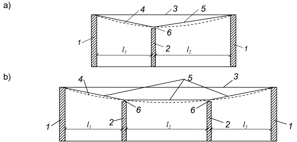
Hình C1 – Sơ đồ xác định các giá trị l, l_1, l_2, l_3 , khi có tường ngăn giữa các tường chịu lực
